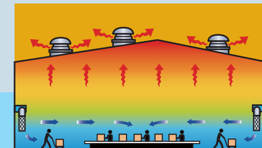
成層空調システム
