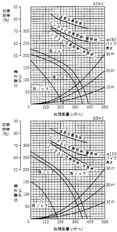
KCI-351(2)J1/KCI-351(2)SJ1
