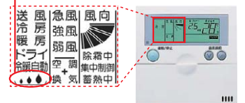
ワイヤードリモコン (PC-AR)
