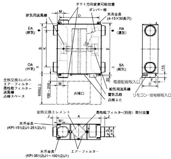
〈KPI-151(2)J1~1001(2)J1〉
