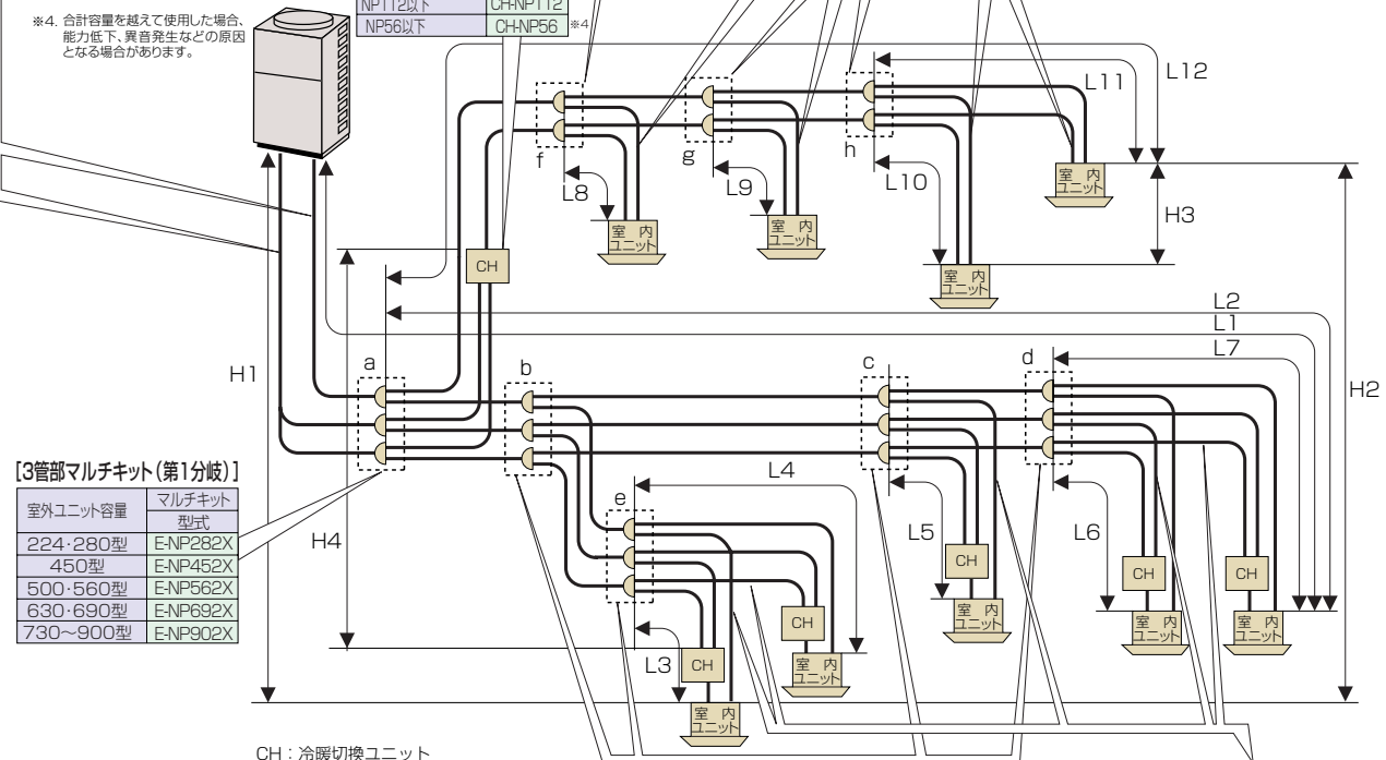
[3管部配管径 (末端分岐～冷暖切換ユニット)]
