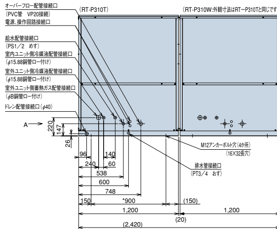
集中ドレンボス (オプション) とアンカーボルト穴の位置
