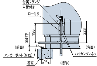
現地施工図 (例)
