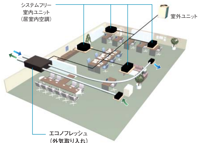
RPIF-AP500K、800K、1000K
