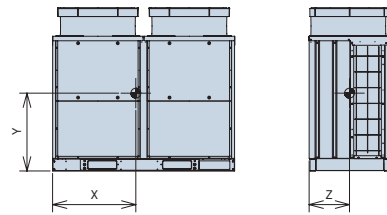
重心位置
