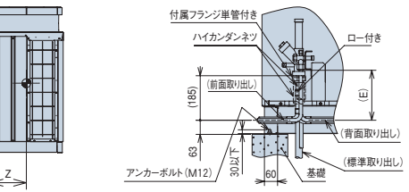
現地施工図 (例)
