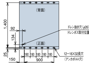
集中ドレンボス (オプション) とアンカーボルト穴の位置
