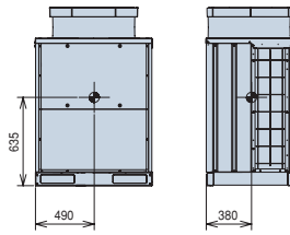
重心位置
