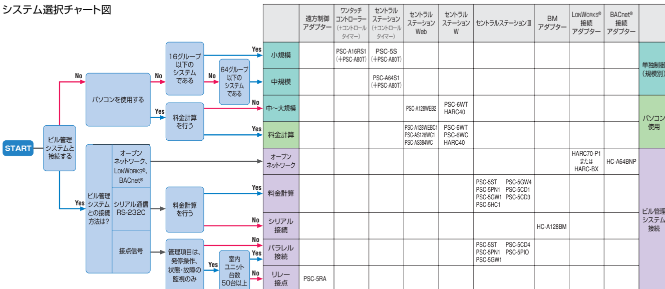
システム選択チャート図
