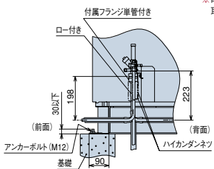
現地施工図 (例)
