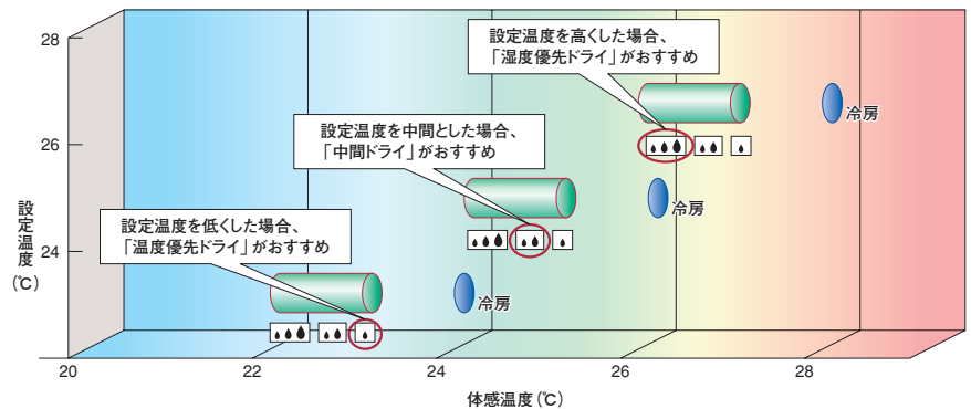
●「爽快除湿運転」による体感温度イメージ図
