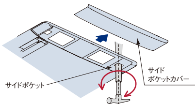
パネル両端のサイドポケットを採用し、パネルを外さずに本体の高さ微調整が容易にできます。
