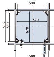
(グリッド天井の場合) (単位:mm)
