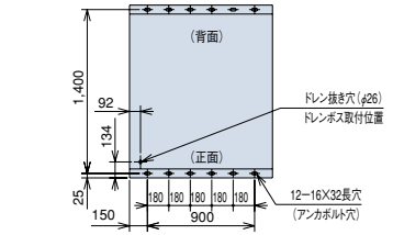
集中ドレンボス (オプション) とアンカーボルト穴の位置
