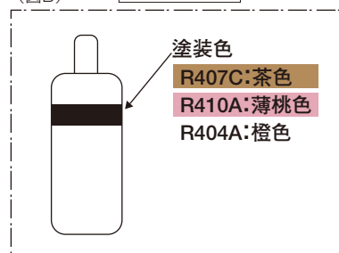
(図B) 冷媒ポンベ
