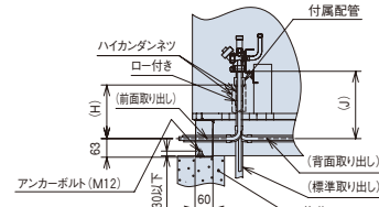
現地施工図 (例)
