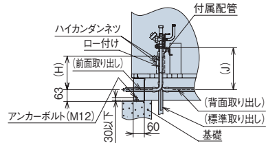
現地施工図(例)
