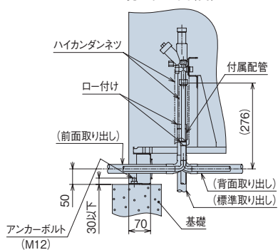
現地施工図(例)
