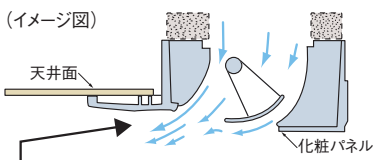
化粧パネルや天井ボードのスマッジングを防ぐため、風の巻き込みに配慮した設計としました。
