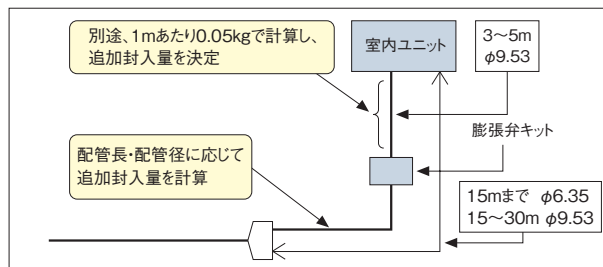
膨張弁キット接続例
