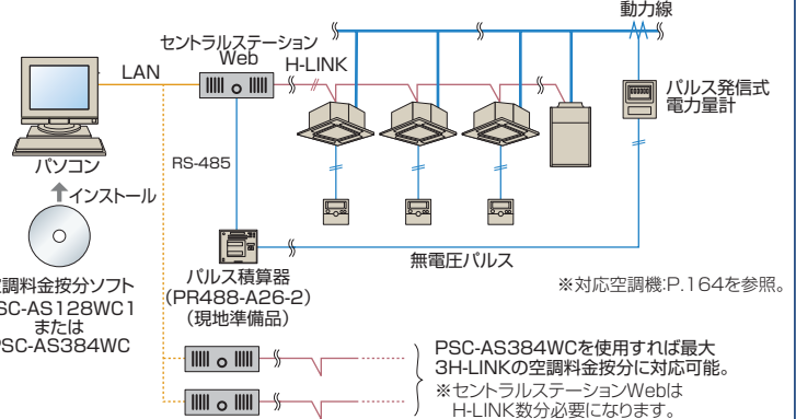
■システム例: 室内/室外が同一電力量計の場合
