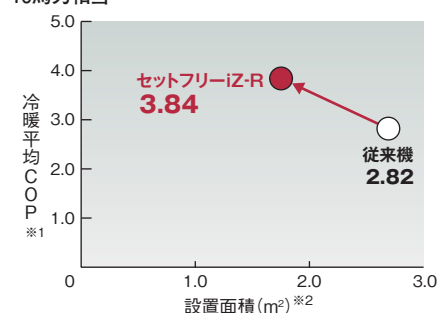
●冷暖平均COPと設置面積の比較（10年前の当社同等従来機との比較）
