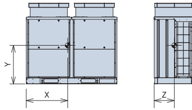
重心位置
