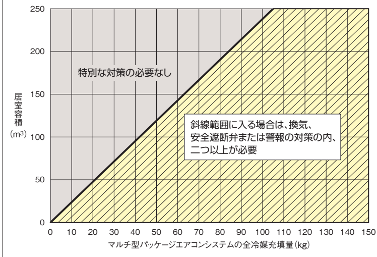
許容冷媒充填量と必要な対策 [R410A冷媒] (地下最下層以外の場合)
