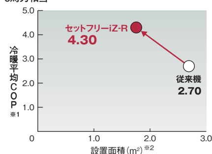
●冷暖平均COPと設置面積の比較（10年前の当社同等従来機との比較）
