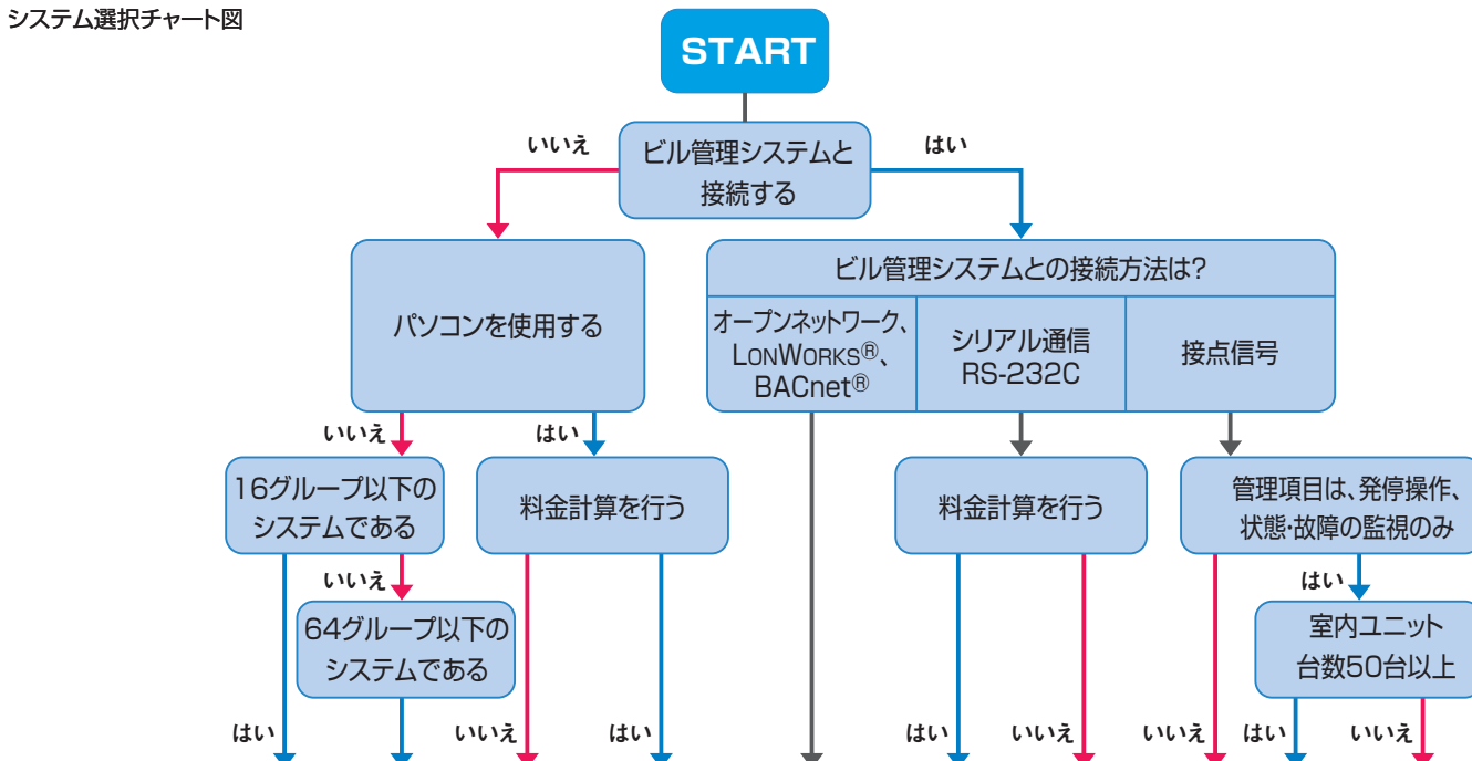
システム選択チャート図
