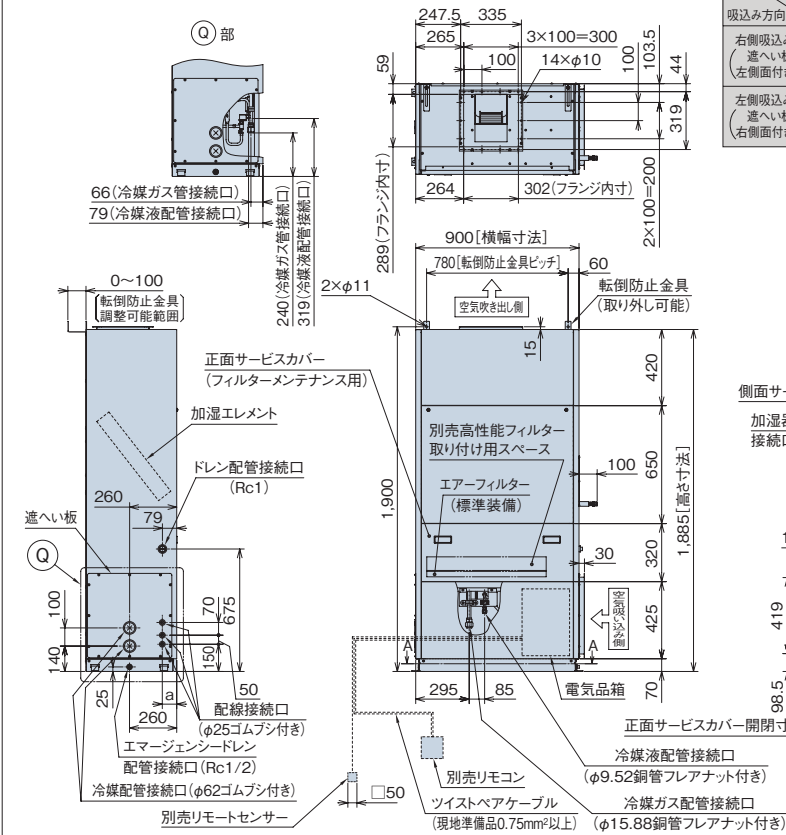
吸い込み方向別寸法表
