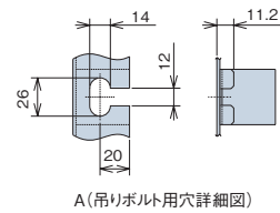
A(吊りボルト用穴詳細図)
