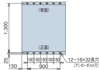
アンカーボルト穴の位置
