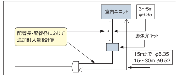
膨張弁キット接続例
