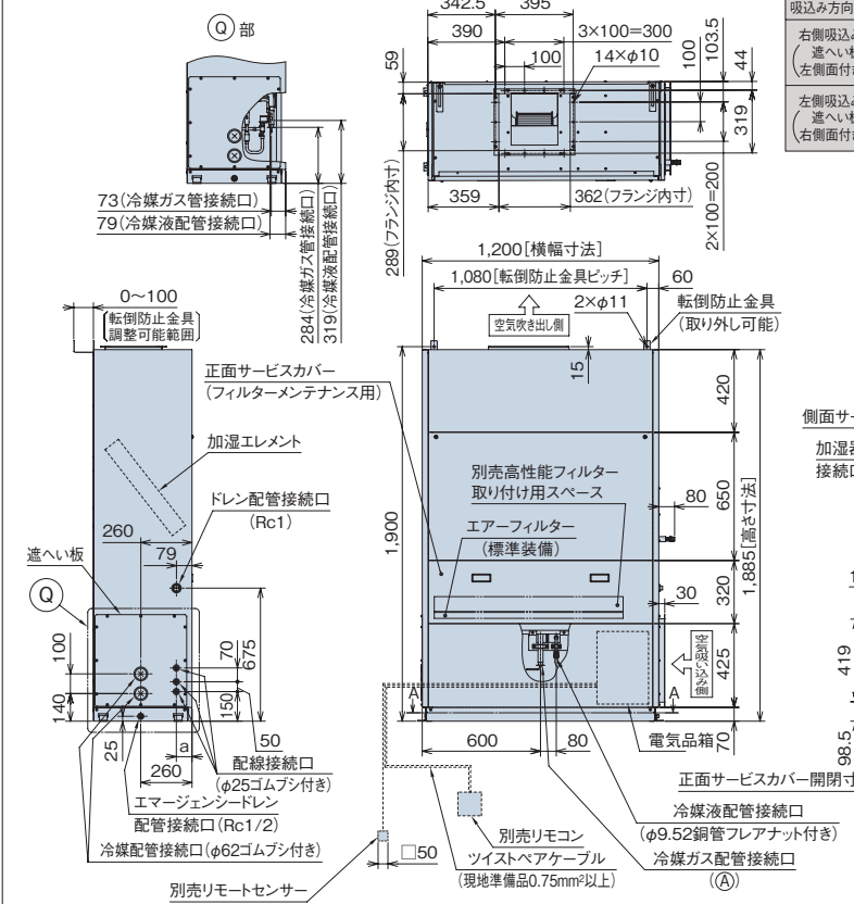
吸い込み方向別寸法表
