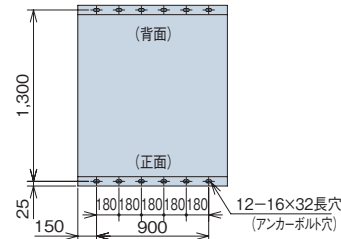
アンカーボルト穴の位置
