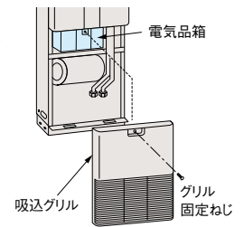
吸込グリル グリル固定ねじ 電気品箱
