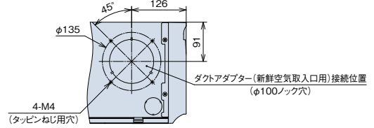
新鮮空気取入キット接続口詳細図
