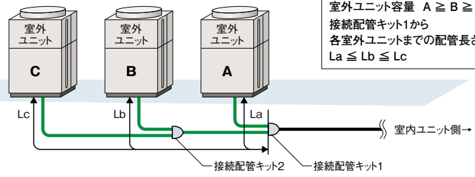
※8 図は室外ユニット正面より見て右方向に配管を引き回した場合を示します。
