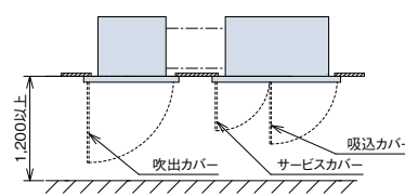
化粧パネルカバー開閉(右側面より見る)
