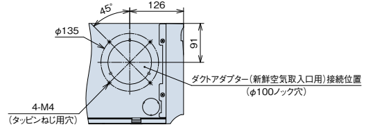
新鮮空気取入口接続口詳細図
