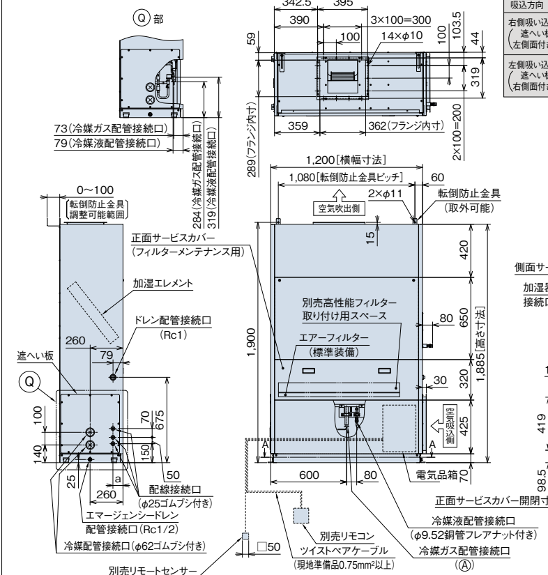
吸込方向別寸法表
