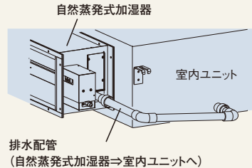
室内ユニット水受けに排水する場合
