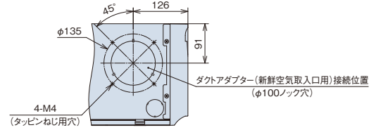
新鮮空気取入キット接続口詳細図
