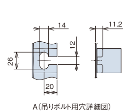
A(吊りボルト用穴詳細図)
