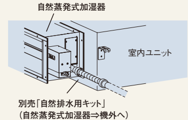
機外に排水する場合※1
