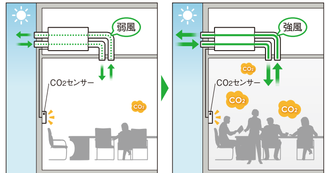
CO 2 濃度が低い場合 弱風 → CO 2 濃度が高い場合 強風
