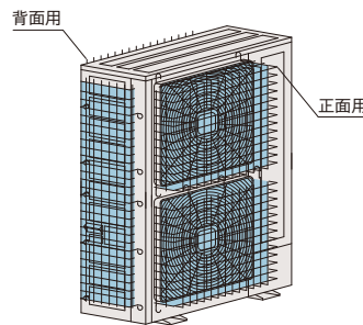
PN-SP10シリーズ 金網ピッチ 50×50mm以下
