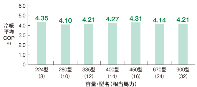
●各容量の冷暖平均COP ※3 [高効率TZシリーズ]
