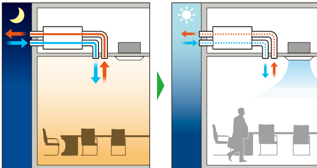
夜中 室内にこもった熱気を排気 → 翌朝 空調機の冷房負荷を低減
