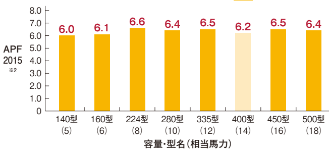
●各容量のAPF2015 ※2 [高効率TGシリーズ]
