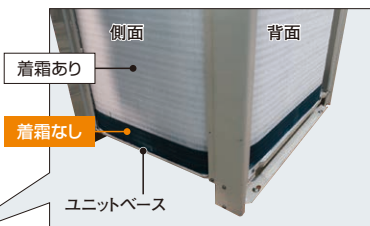
外気温度：2°CDB/1°CWBの暖房運転時。製造元の恒温試験室にて撮影。
