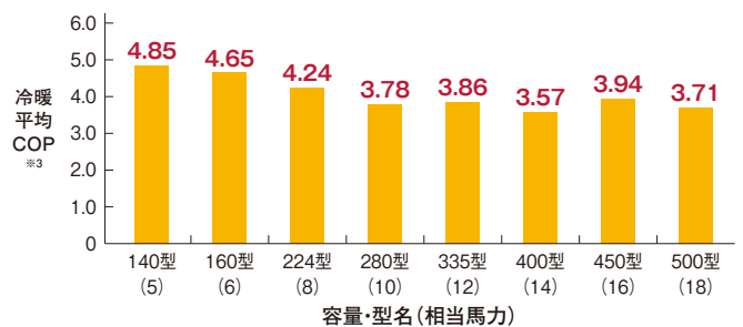
●各容量の冷暖平均COP ※3 [高効率TGシリーズ]
