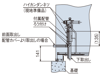
現地配管施工図(例)
