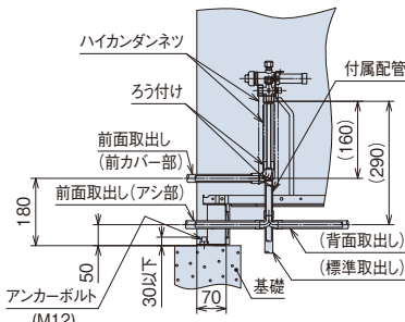
現地施工図(例)
