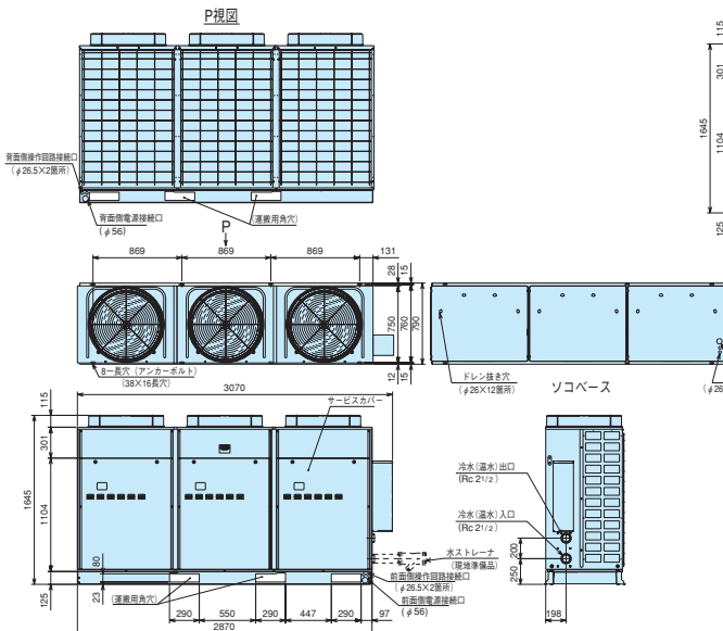
空冷式中温用スクロールチラーユニット (RCUP750AM2)
