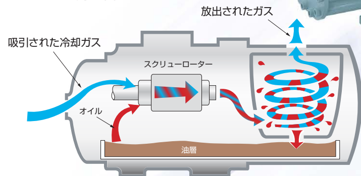
サイクロン式原理図
