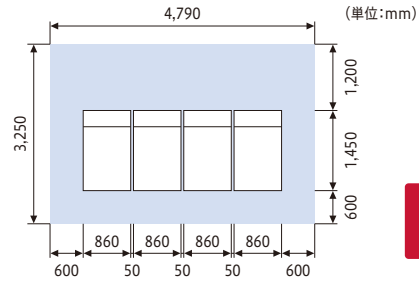
■RCF1320WVTC[40馬力相当機]の4台連続設置例
