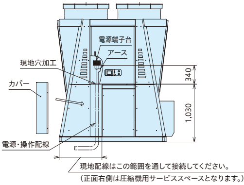
【電源・操作配線接続口詳細】
