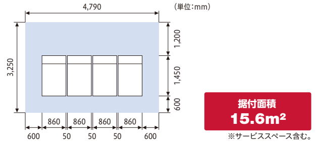
■RCF1320WVTC[40馬力相当機]の4台連続設置例
