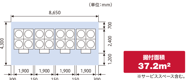
■RHF1500AV1 [50馬力相当機]標準仕様の4台連続設置例
