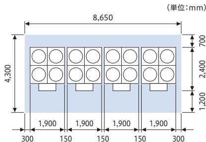
■RHF1500AV1 [50馬力相当機]標準仕様の4台連続設置例
