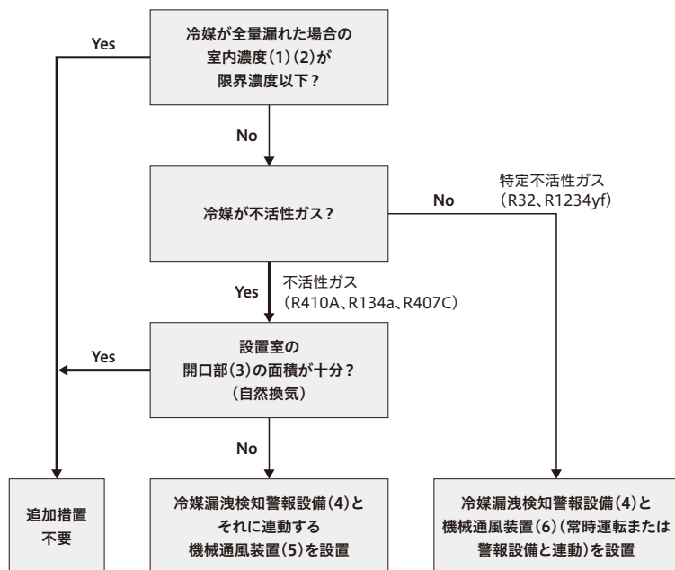
■冷媒漏洩に対する安全対策フローチャート
