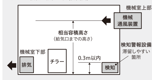
●チラー機械室設置の例(側面図)
