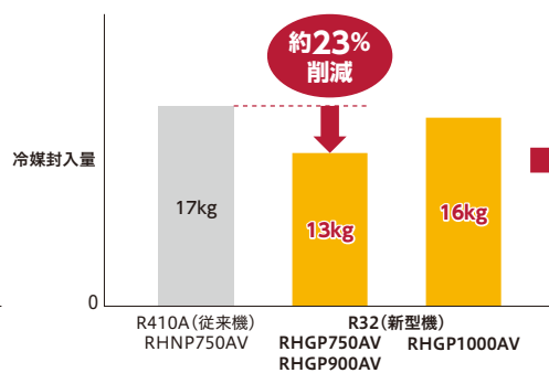
冷媒封入量
