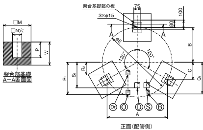
基礎寸法図
