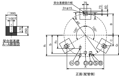
基礎寸法図
