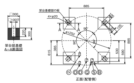
基礎寸法図
