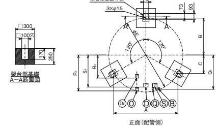
基礎寸法図
