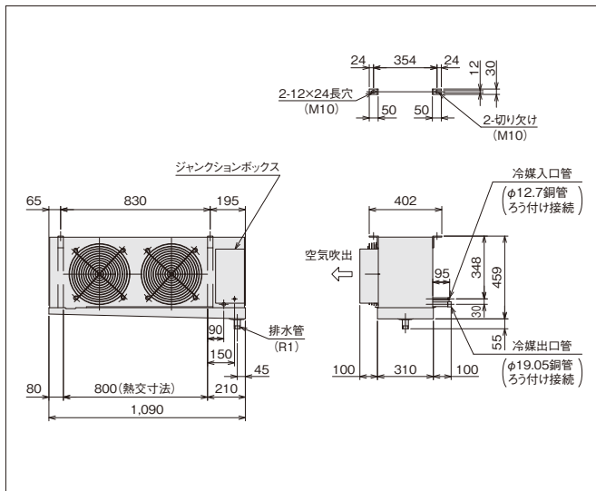
US-T3H1 / US-T3MH1 / US-T3LH1 (単位:mm)
