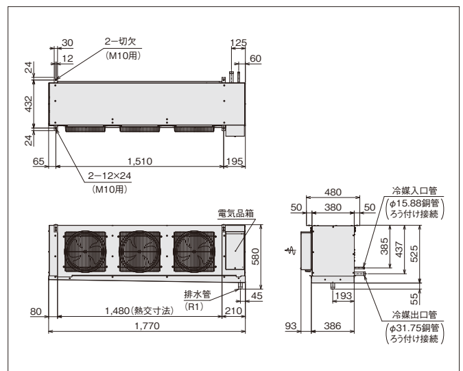
US-T6H / US-T6MH / US-T6LH (単位:mm)
