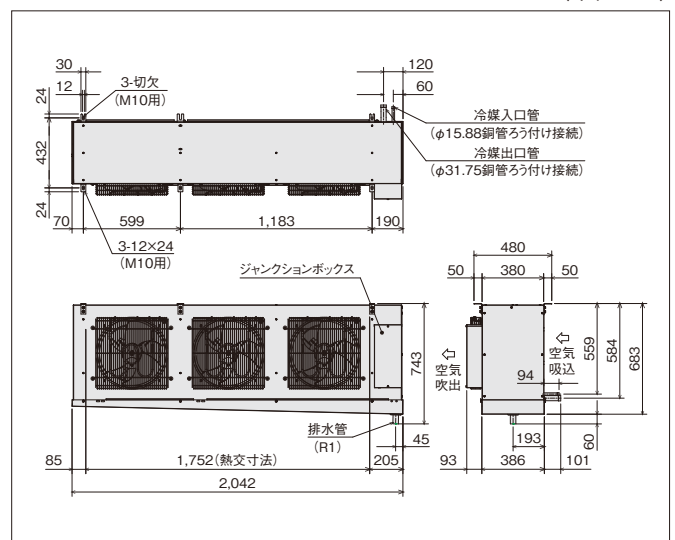
US-T10H1 / US-T10MH1 / US-T10LH1 (単位:mm)
