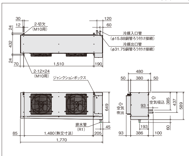
US-T8H1 / US-T8MH1 / US-T8LH1 (単位:mm)
