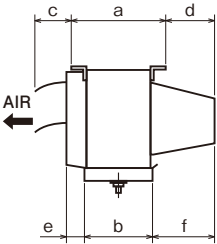
寸法対応図
