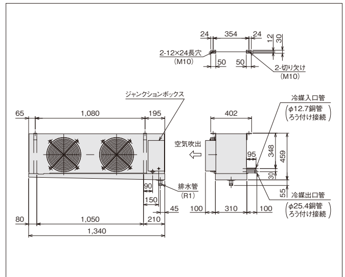
US-T4H1 / US-T4MH1 / US-T4LH1 (単位:mm)
