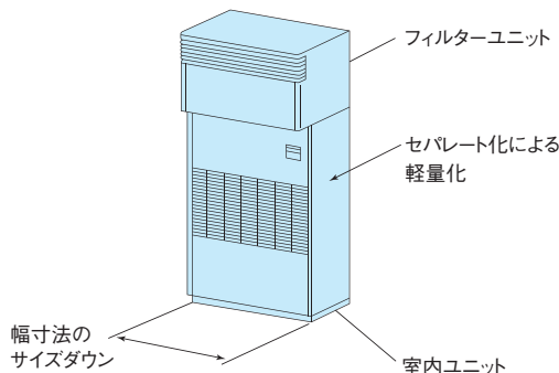
室内ユニットの仕様比較(冷暖兼用・直吹型の場合)
