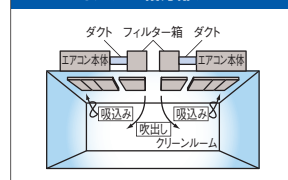
フィルター箱分離タイプ
