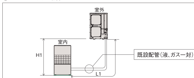
③ 800型の場合
