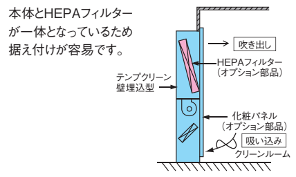
直吹出タイプ(HEPAフィルター付)
