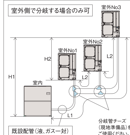
③ 800型の場合
