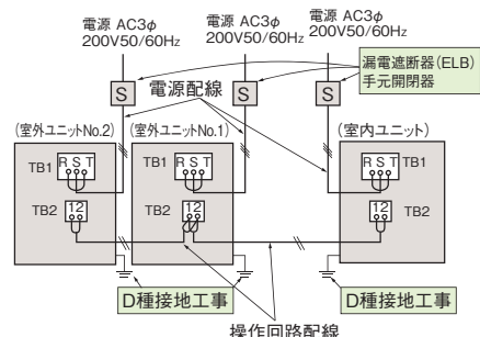
床置セパレート型の場合
