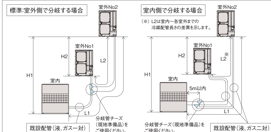
② 450～630型の場合
