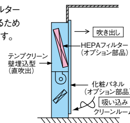
直吹出タイプ(HEPAフィルター付)
