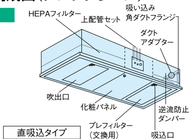
直吸込タイプ
