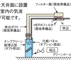
ダクト吹出タイプ(フィルター箱分離)
