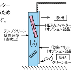
直吹出タイプ(HEPAフィルター付)
