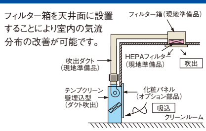
ダクト吹出タイプ(フィルター箱分離)
