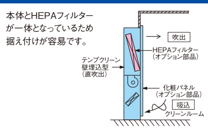
直吹出タイプ(HEPAフィルター付)
