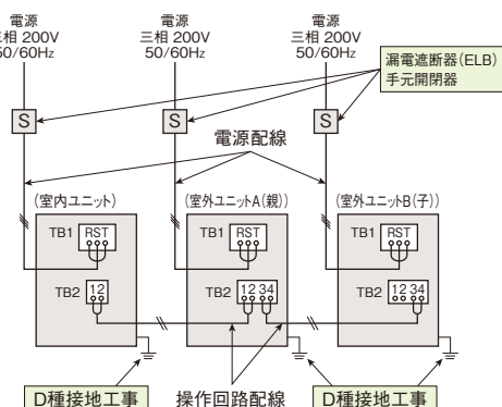
床置セパレート型の場合の一例
