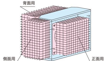
アクティブフィルター (室外ユニット取り付け型)
