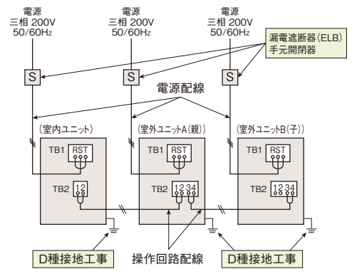
床置セパレート型の場合の一例
