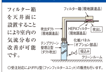
ダクト吹出タイプ(フィルター箱分離)
