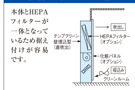
直吹出タイプ(HEPAフィルター付)
