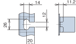
A(吊りボルト用穴詳細図)
