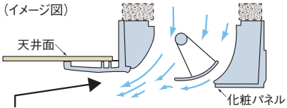
(イメージ図) 化粧パネルや天井ボードのスマッシングを抑制するため、風の巻き込みに配慮した設計としました。
