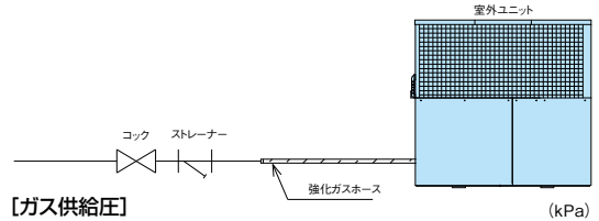
【ガス供給圧】
