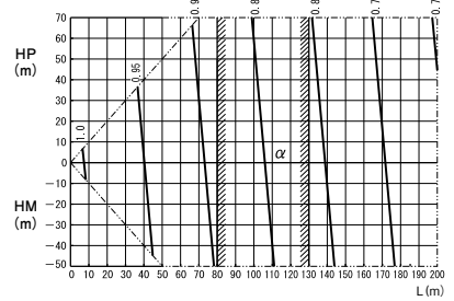
配管長スイッチ : L設定
