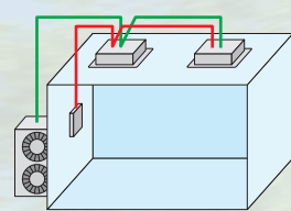
個別制御 (運転ON・OFF同時) サーモON・OFF個別
