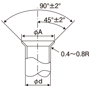
フレア形状
