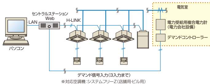
■システム例：デマンドコントローラーを接続する場合
