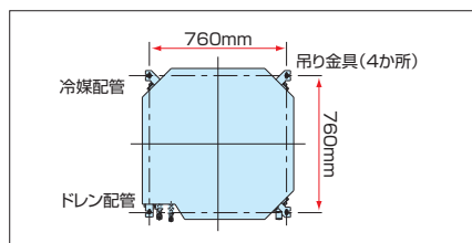
丸ダクト接続時
