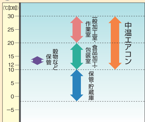
● 生産・加工・保管に対応する中温エアコンの環境製造室温度
