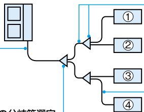
第1分岐の分岐管選定
