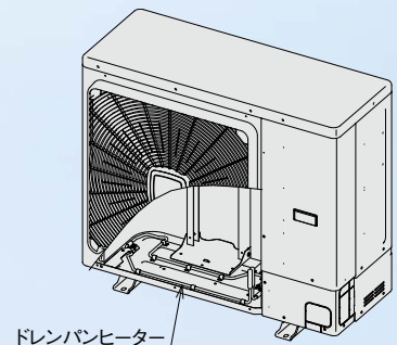
*ドレンパンヒーターは防雪フード(深形フード)一式(吹出口・背面吸込口・左吸込口)と併用して使用してください。
