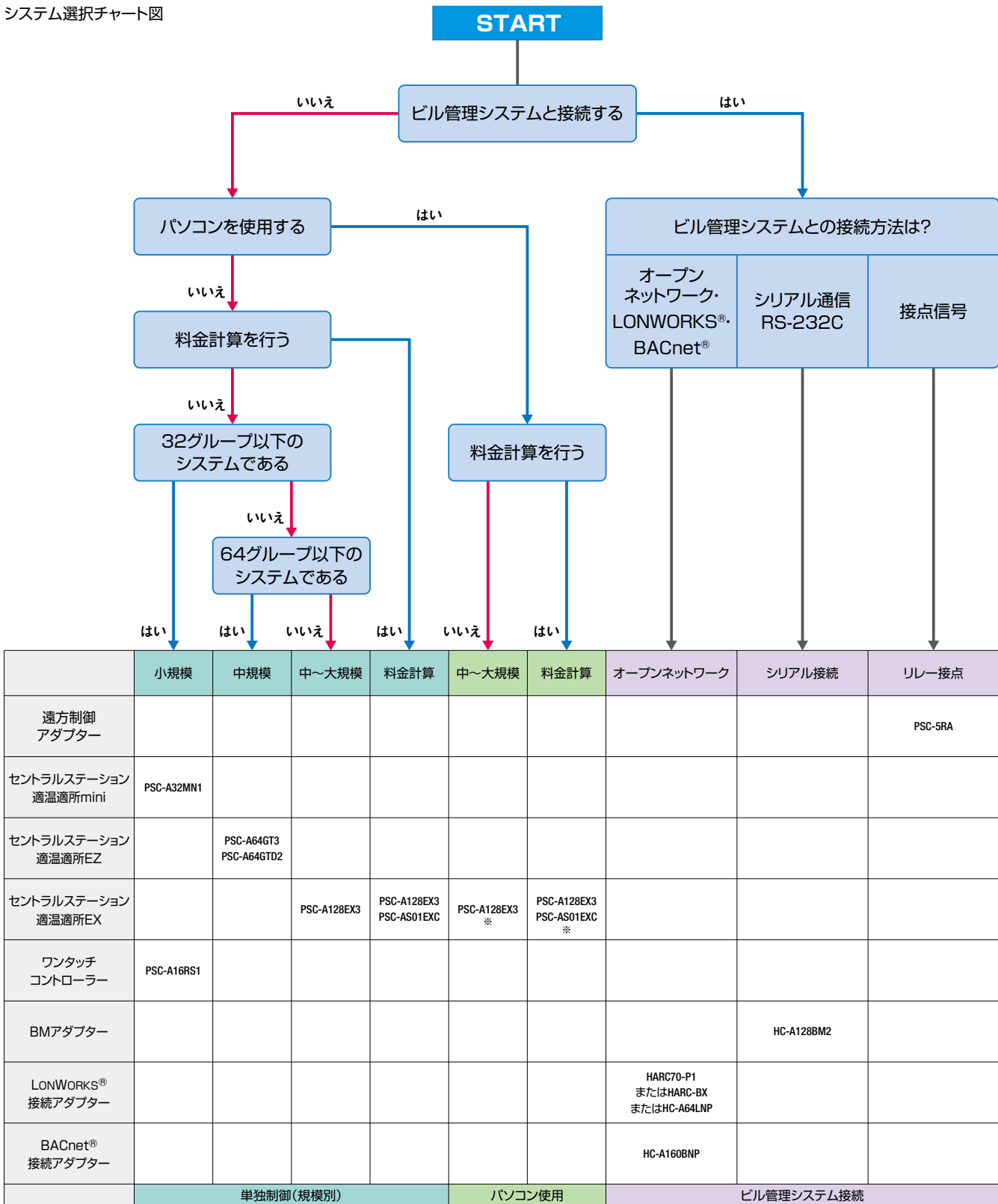
システム選択チャート図
