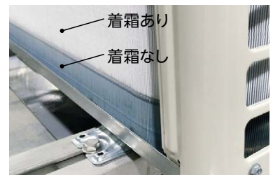
外気温度2°CDB/1°CWBの暖房運転時。製造元の試験室で撮影。
