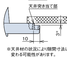
S部詳細
