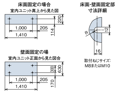
床面・壁面固定部寸法
