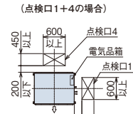
■上面図 (点検口1+4の場合)
