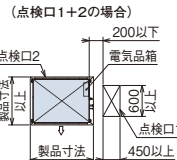
■上面図 (点検口1+2の場合)
