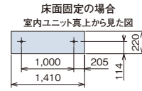
床面・壁面固定部寸法
