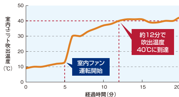
■フィールド評価機 寒さ知らず: RAS-AP280DN
