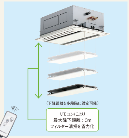
昇降専用ワイヤレスリモコン(オプション)
