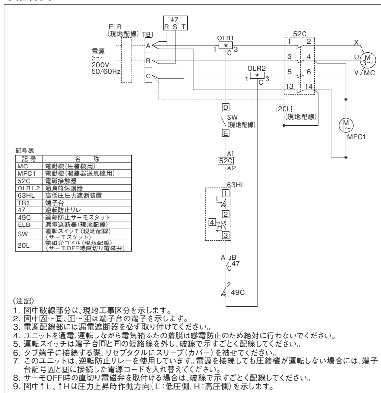
●配線図
