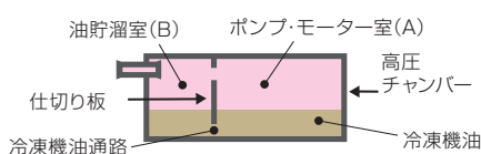
差圧油面確保構造 (横型スクロール圧縮機)
