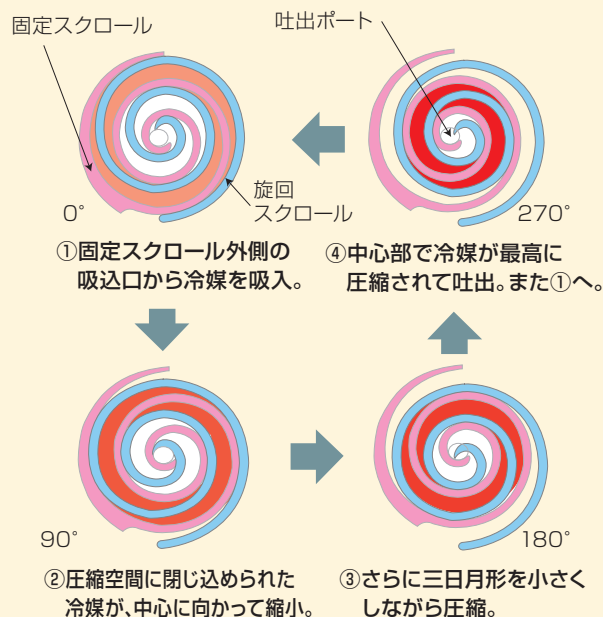
スクロール圧縮機の圧縮工程
