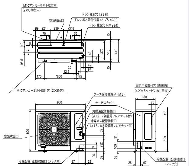
室外ユニット標準寸法図
