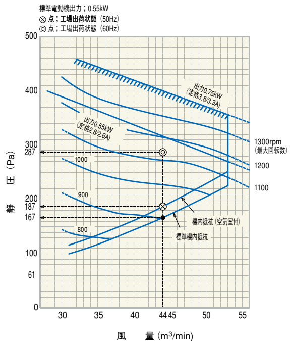
送風機特性曲線
