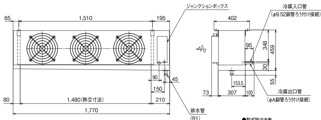
●型式別寸法表
