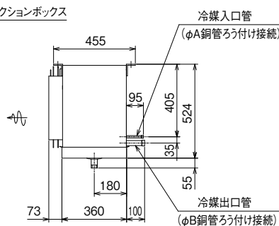
●型式別寸法表
