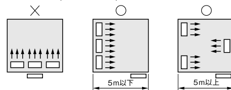
ウォークインタイプ 配置例
