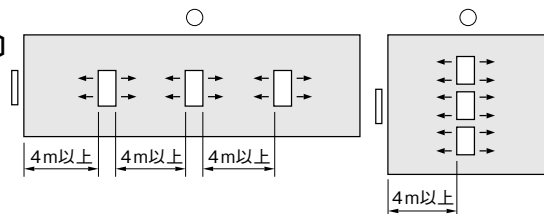
低風量タイプ 配置例
