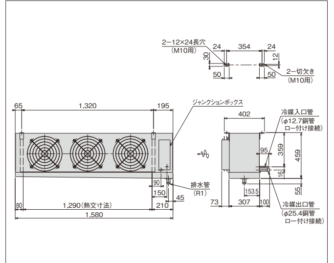
US-R5H1 / US-R5MH1 (単位:mm)
