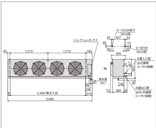
US-R16H1 / US-R16MH1 / US-R16LH1 (単位:mm)
