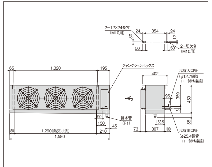
US-R5H1 / US-R5MH1 / US-R5LH1 (単位:mm)
