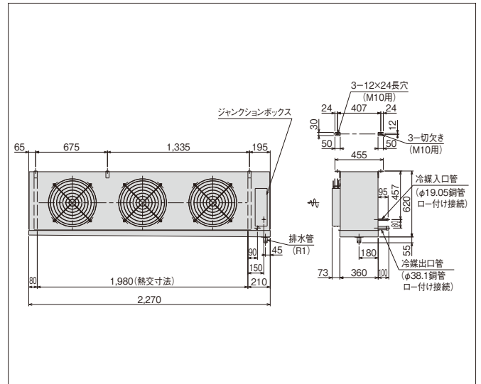
US-R13H1 / US-R13MH1 / US-R13LH1 (単位:mm)
