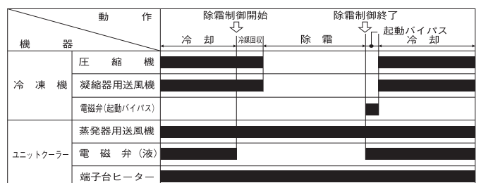
オフサイクル除霜中の各機器の動作
