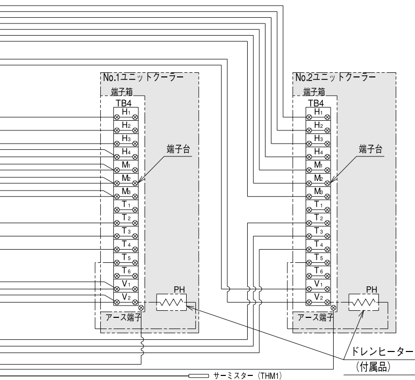
■配線および遮断器容量
