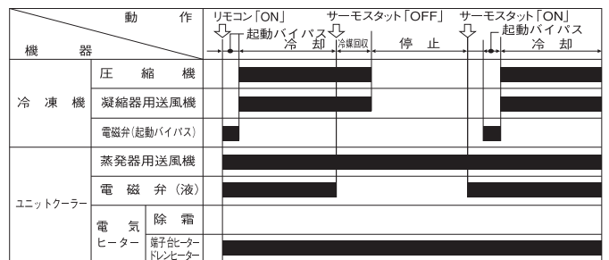
冷却運転中の各機器の動作
