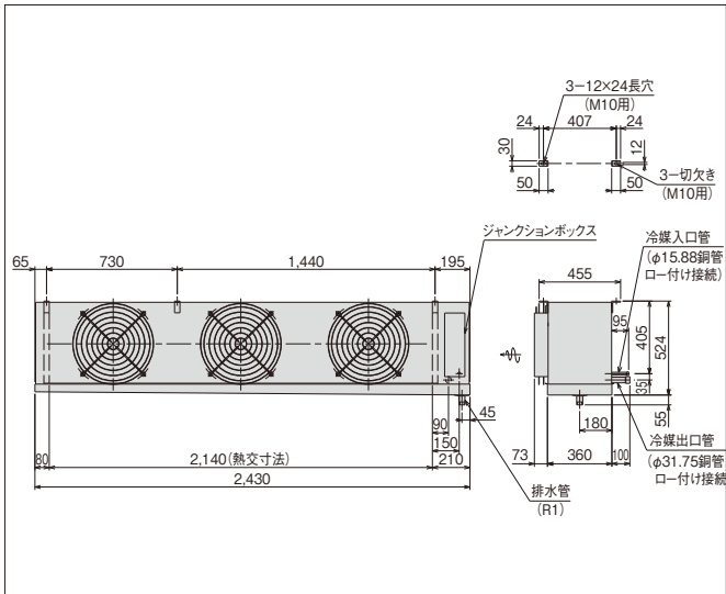
US-R10H1 / US-R10MH1 / US-R10LH1 (単位:mm)
