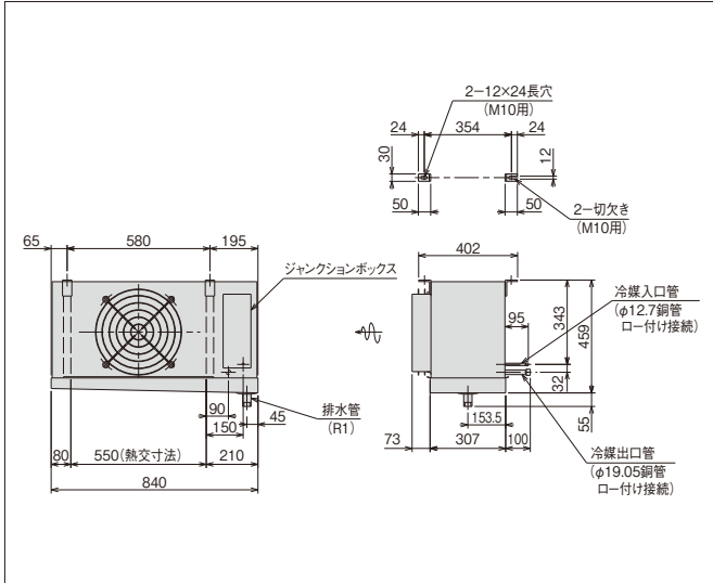
US-R2H1 / US-R2MH1 / US-R2LH1 (単位:mm)
