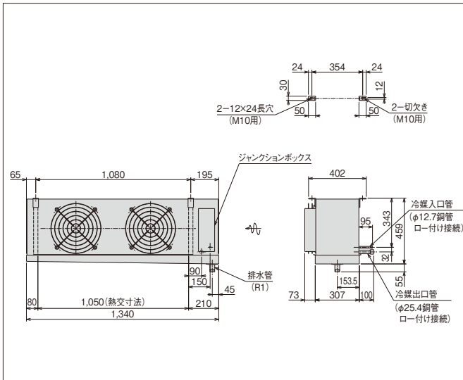
US-R4H1 / US-R4MH1 / US-R4LH1 (単位:mm)
