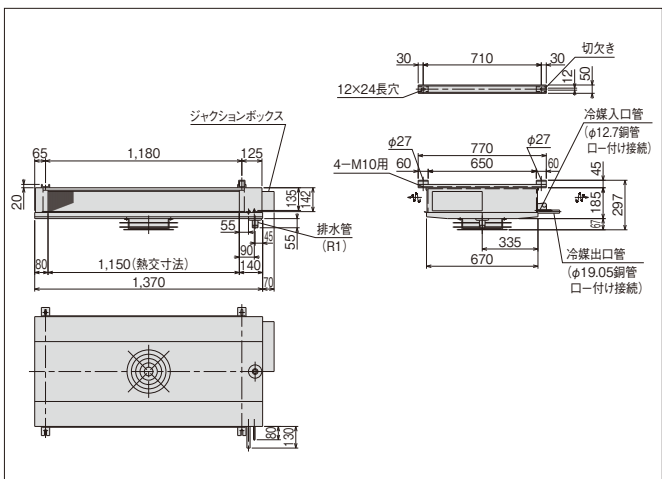
US-R2HT1 / US-R2MHT1 (単位:mm)
