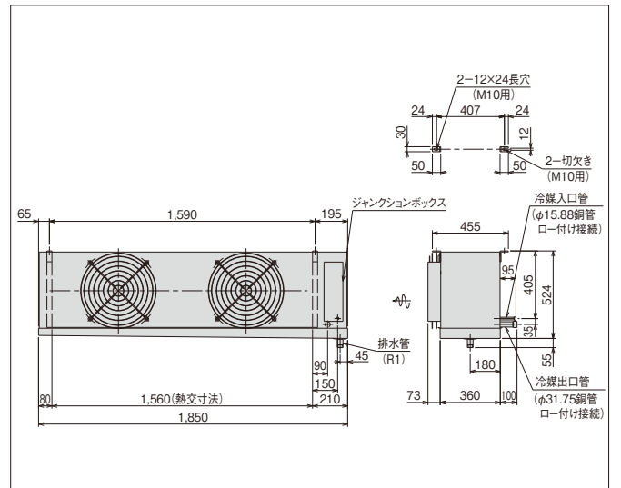
US-R8H1 / US-R8MH1 / US-R8LH1 (単位:mm)
