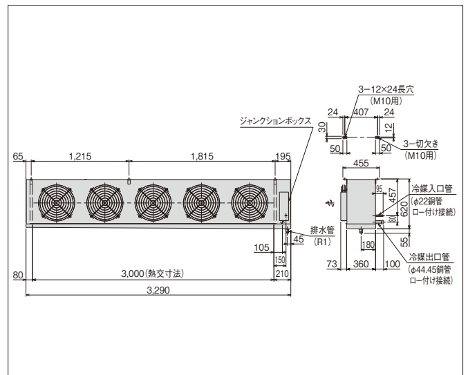
US-R20LH1 (単位:mm)
