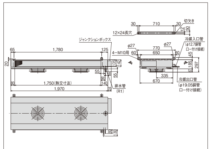
US-R3HT1 / US-R3MHT1 (単位:mm)
