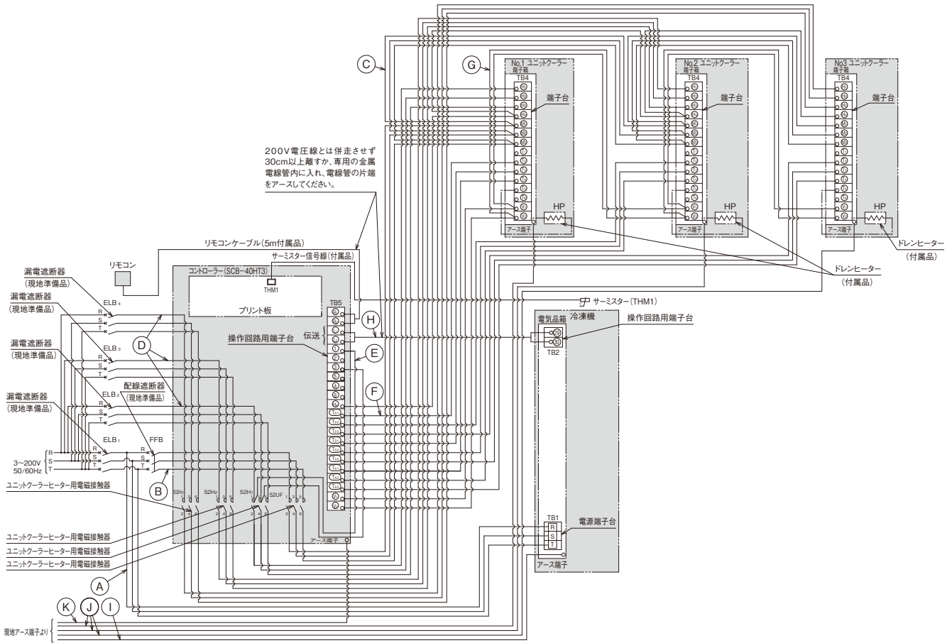
■配線および遮断器容量
