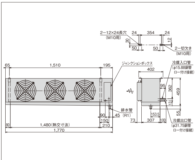
US-R6H1 / US-R6MH1 / US-R6LH1 (単位:mm)
