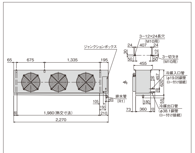
US-R13H1 / US-R13MH1 / US-R13LH1 (単位:mm)
