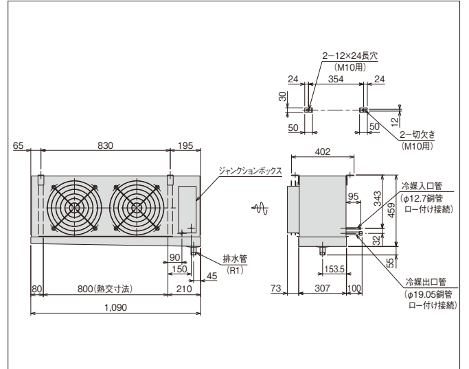
US-R3H1 / US-R3MH1 / US-R3LH1 (単位:mm)
