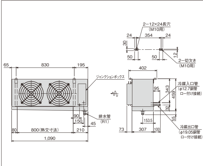
US-R3H1 / US-R3MH1 / US-R3LH1 (単位:mm)
