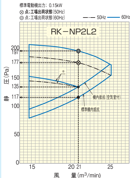
送風機特性曲線
