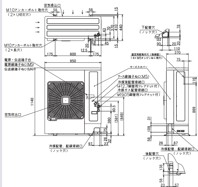
室外ユニット寸法図 (RAS-GP5T)
