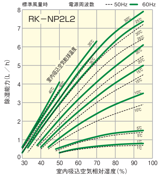
除湿能力特性
