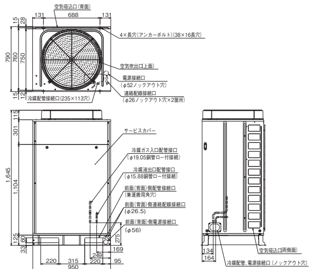
室外ユニット寸法図
