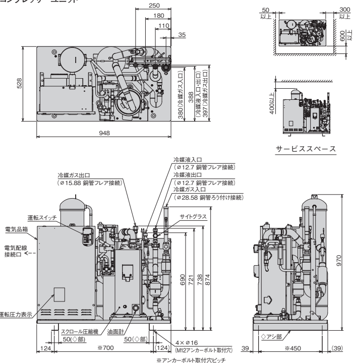
(写真はKX-T8CVです) (単位:mm)
