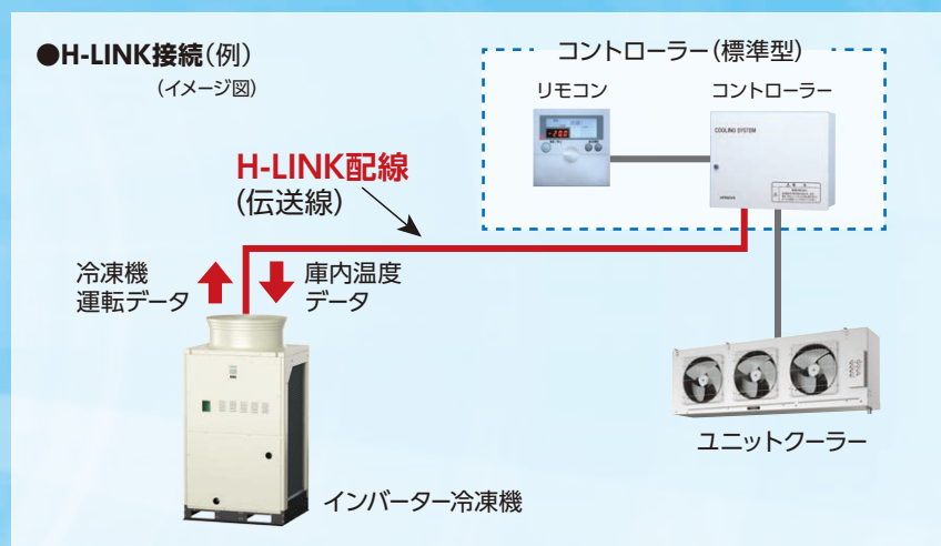
標準型コントローラーまたは 高機能型コントローラー
