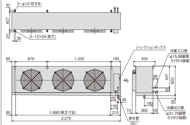
US-N13H2/US-N13MH2/US-N13LH2 (単位:mm)
