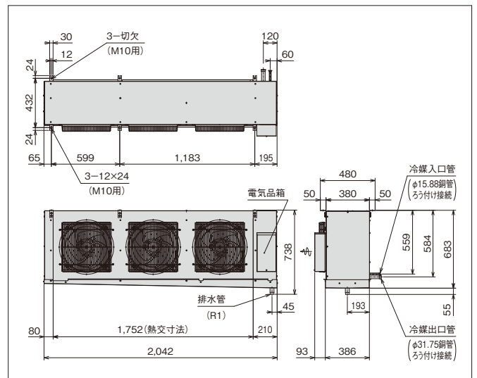
US-T10H / US-T10MH / US-T10LH (単位:mm)
